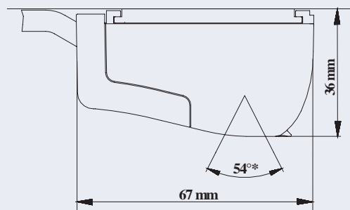
Plafonra szerelés
