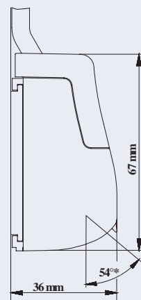
Falra szerelés
